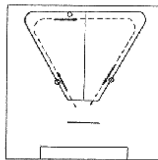
Рис. 9. 3-я фаза - оценка движений лошади на тыгу
